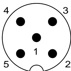
Würfel-Stecker
